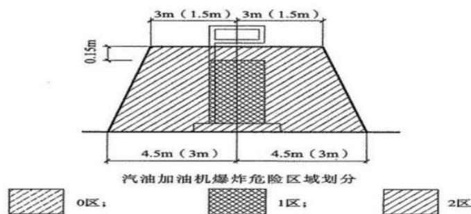
图 3.6-1 汽油加油机爆炸危险区域划分图
